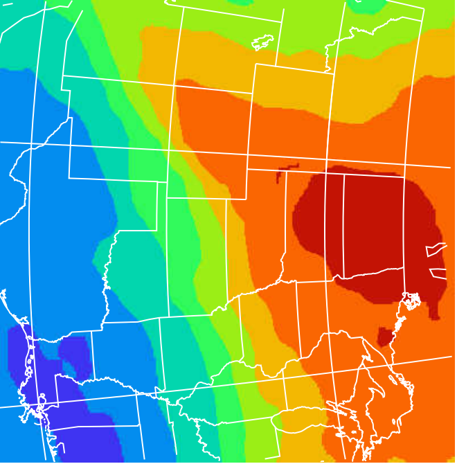
TOMS 12/4/96
