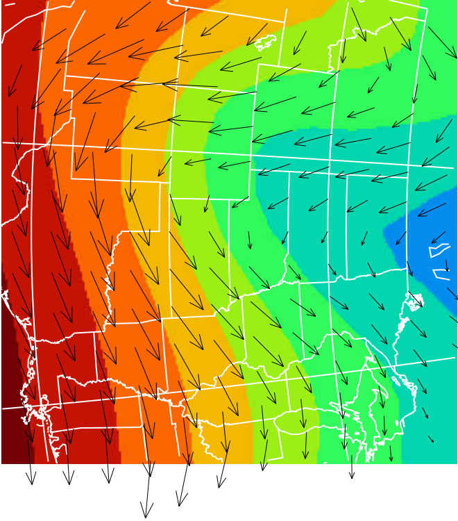
500 hPa Z 12/4/96
